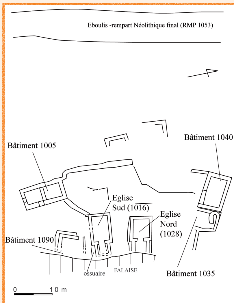
Illustration 4 : plan général de la première enceinte néolithique et des deux église du haut Moyen Age parmi les structures de la fin du XIII ème siècle
